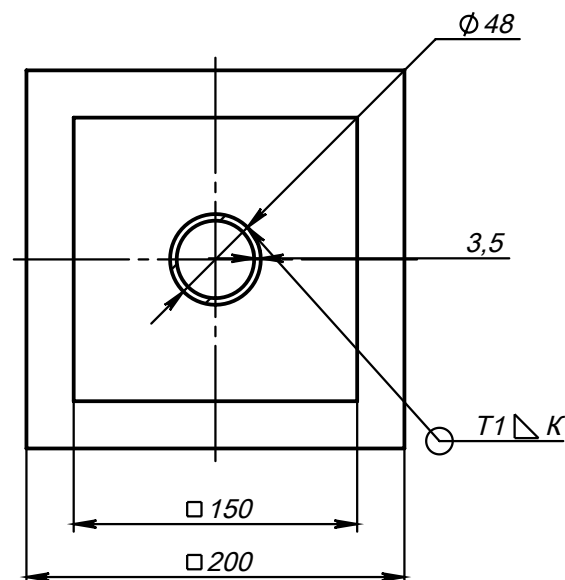
A-A
