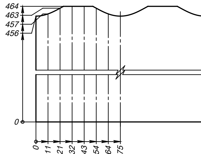
Поз.4 (Труба) развертка 1:2
